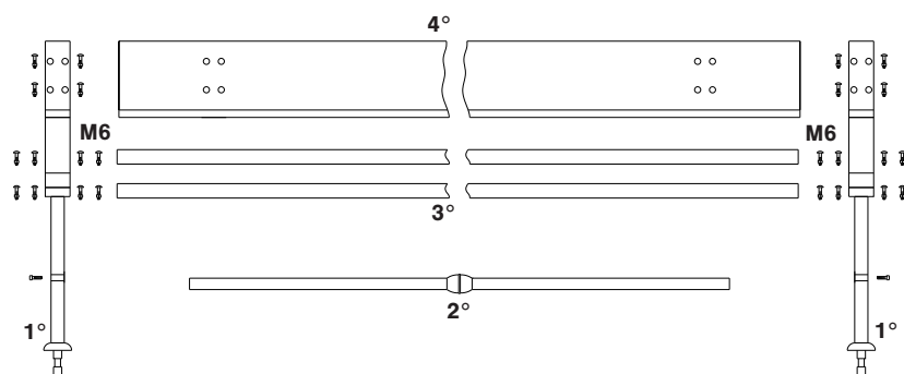
Vue éclatée
